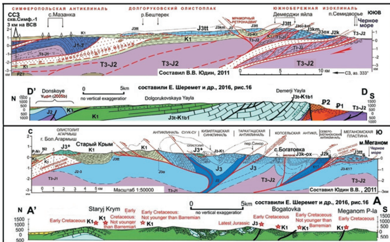
Рис. 2. Сравнение геологических разрезов [13] с разрезами, составленными по тем же районам в статье [22, рис. 15]
