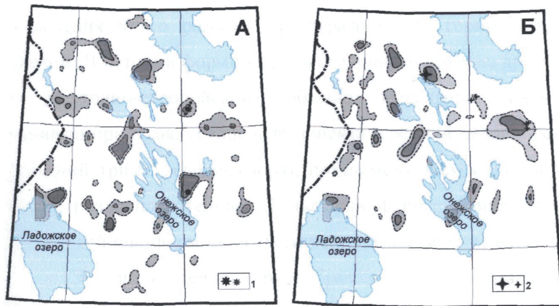
Рис. 6.2.10. Размещение перспективных участков для локализации руд: А — меди и никеля в связи с расслоенными интрузиями нижнего протерозоя; Б — золота в фундаментах древних платформ в пределах Ладожско-Онежской площади.
