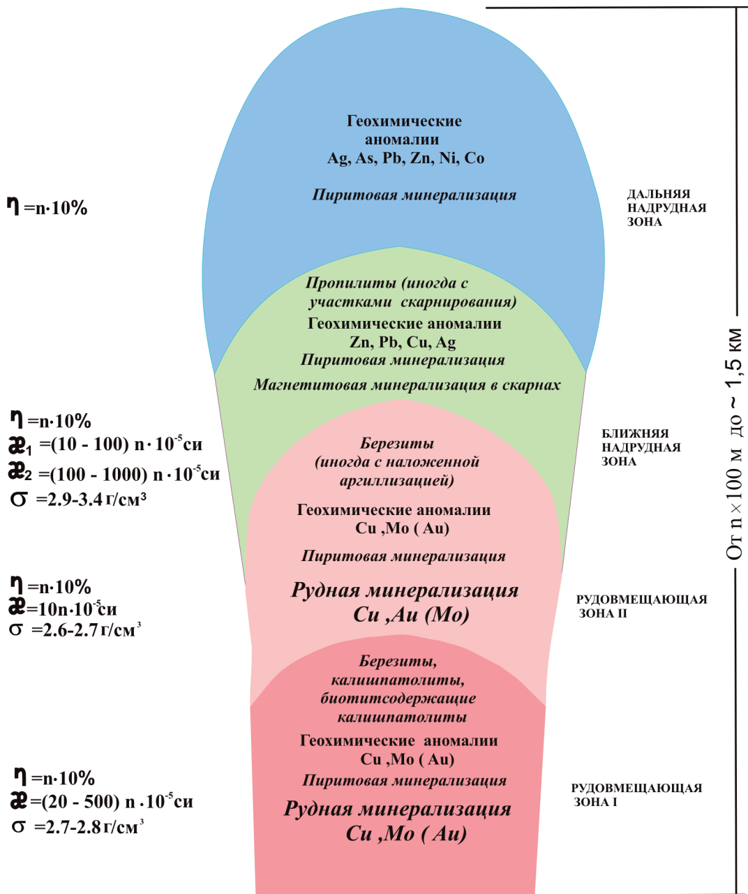
Рис. 3.4. Модель рудно-геохимической, гидротермально-метасоматической и петрофизической зональности молибден-меднопорфировых месторождений березитового типа. Составил М. Л. Сахновский.
