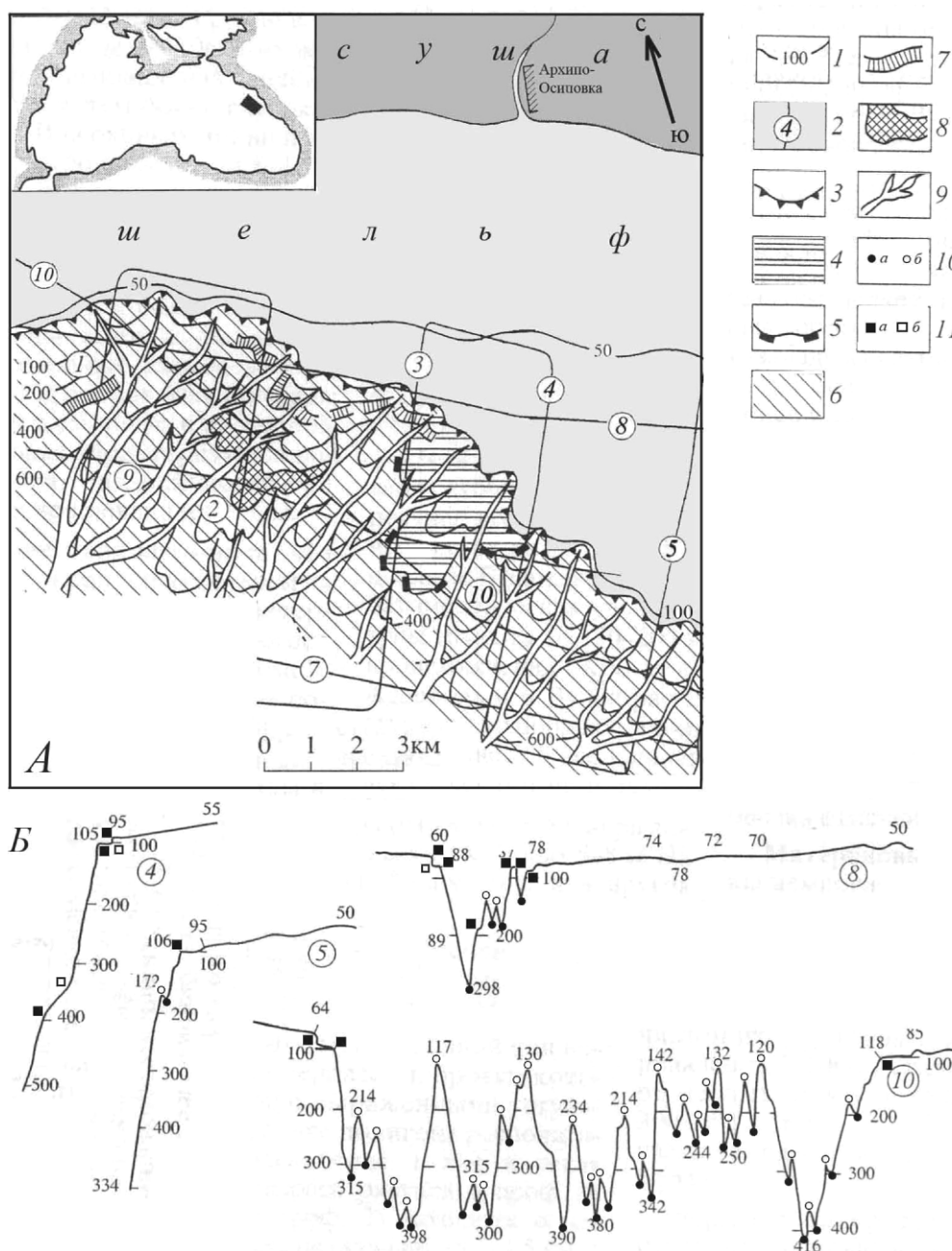
Рис. 6. Обзорная схема (А) и характерные профили дна (Б) Черного моря по данным эхолотирования (по [7] с изменениями). Поперечные (4, 5) и продольные (8, 10) профили выявляют разные особенности морфологии дна.
